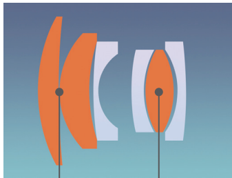
镜片结构5组6片
